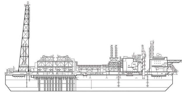
Le FPSO mesure 270 m de long et 61,4 m de haut.
