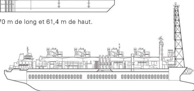
Le FLNG mesure 294 m de long.
